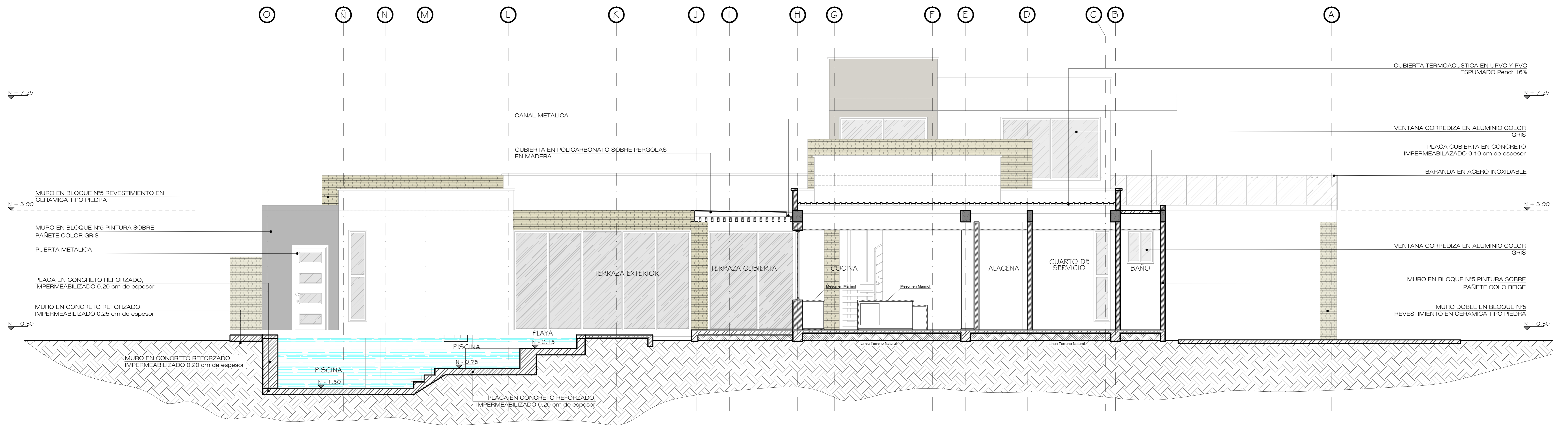
CORTE D - D ESC 1:50
