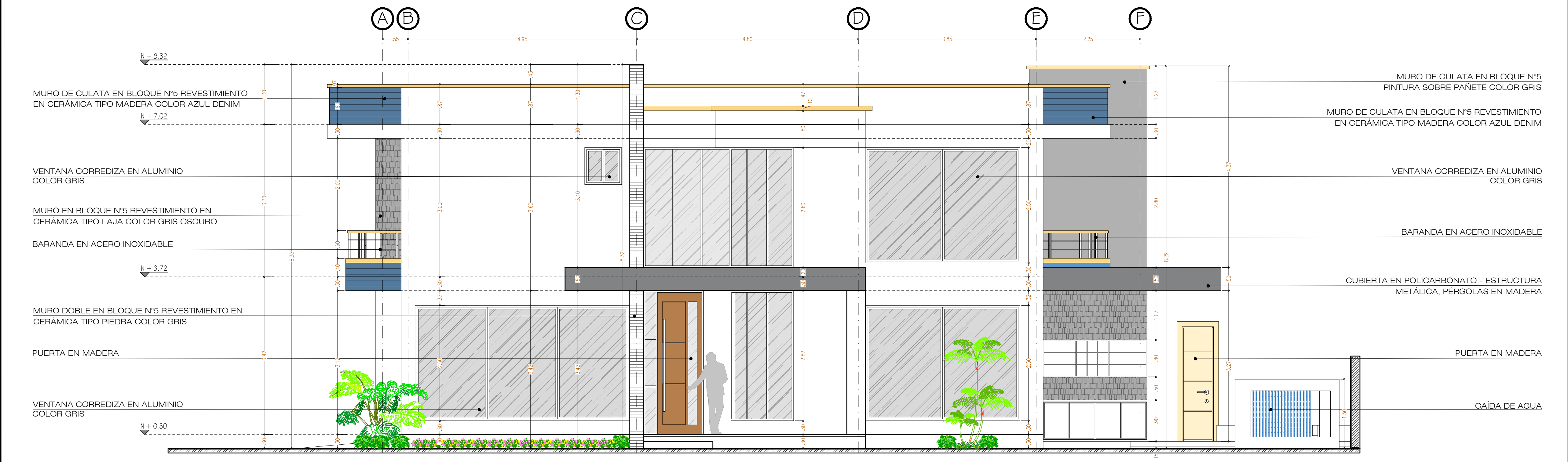
FACHADA PRINCIPAL__ESC_1:50
