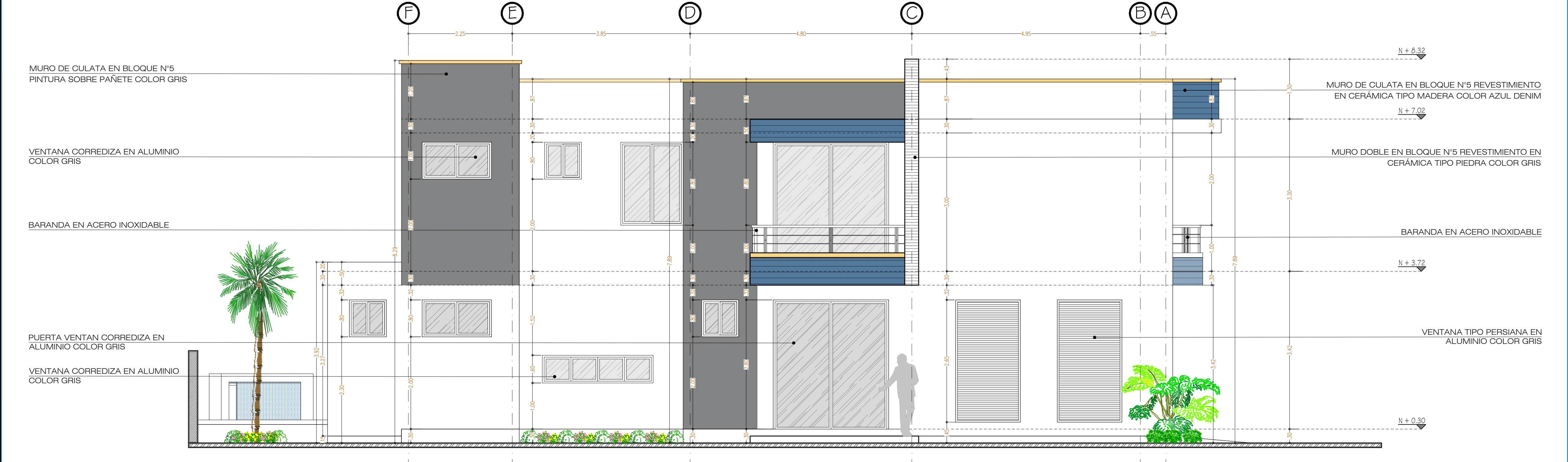
FACHADA POSTERIOR__ESC_1:50
